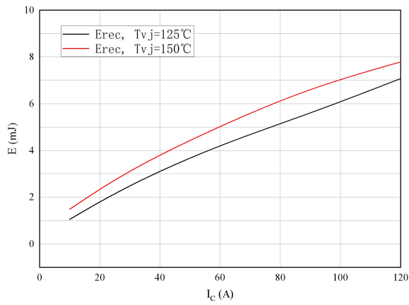
图 7. 开关损耗 二极管 Figure 7. Switching losses of Diode RGon=10Ω, VCE=600V
