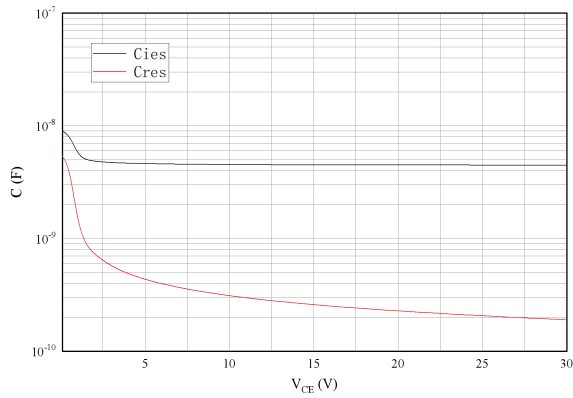
图 9. 电容特性 Figure 9. Capacitance characteristic
